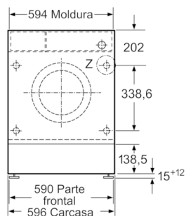
Detalle Z
