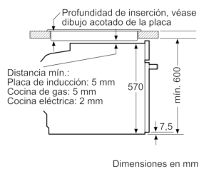
Montaje con una placa.
