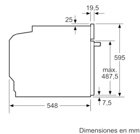
Montaje con una placa.
